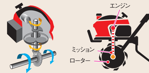
エンジンの下にミッションと耕うん爪を収める「タテ型」のコンパクト設計
