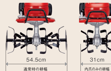
通常時の耕幅
